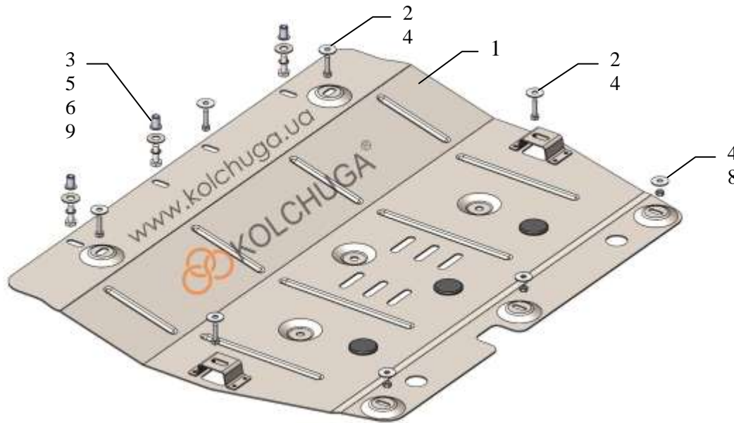
Схема збірки захиста.
