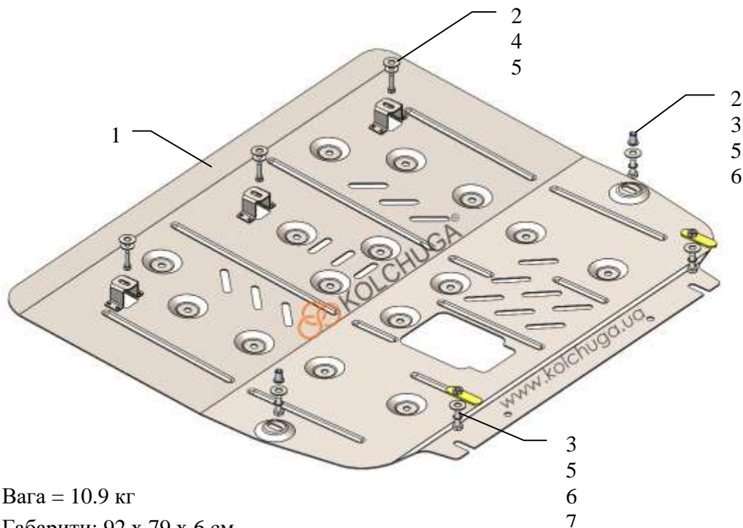
Схема захисту.
