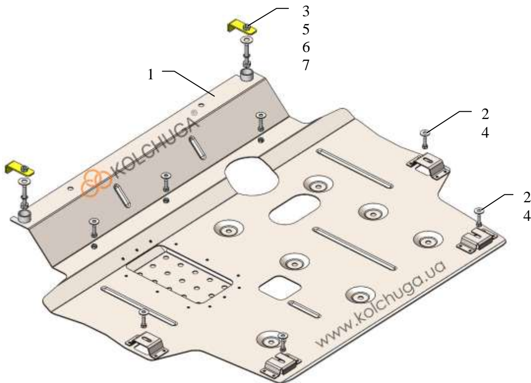
Схема захисту.
