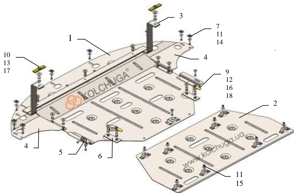
Схема захисту.
