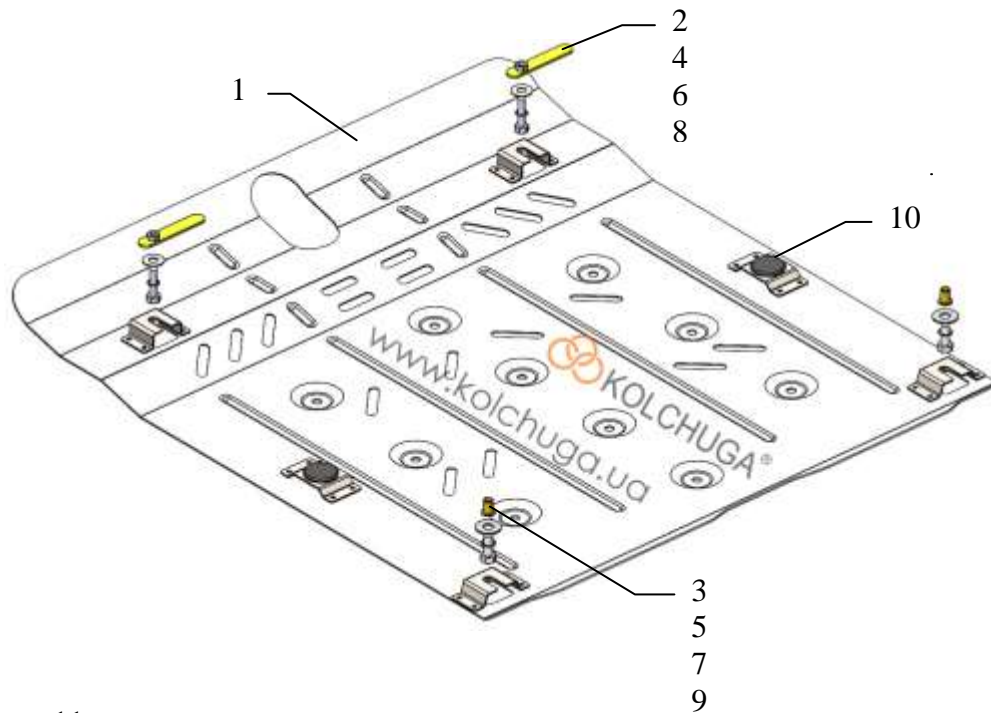
Схема захисту.
