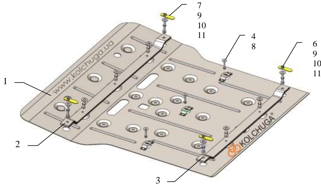
Схема захисту.
