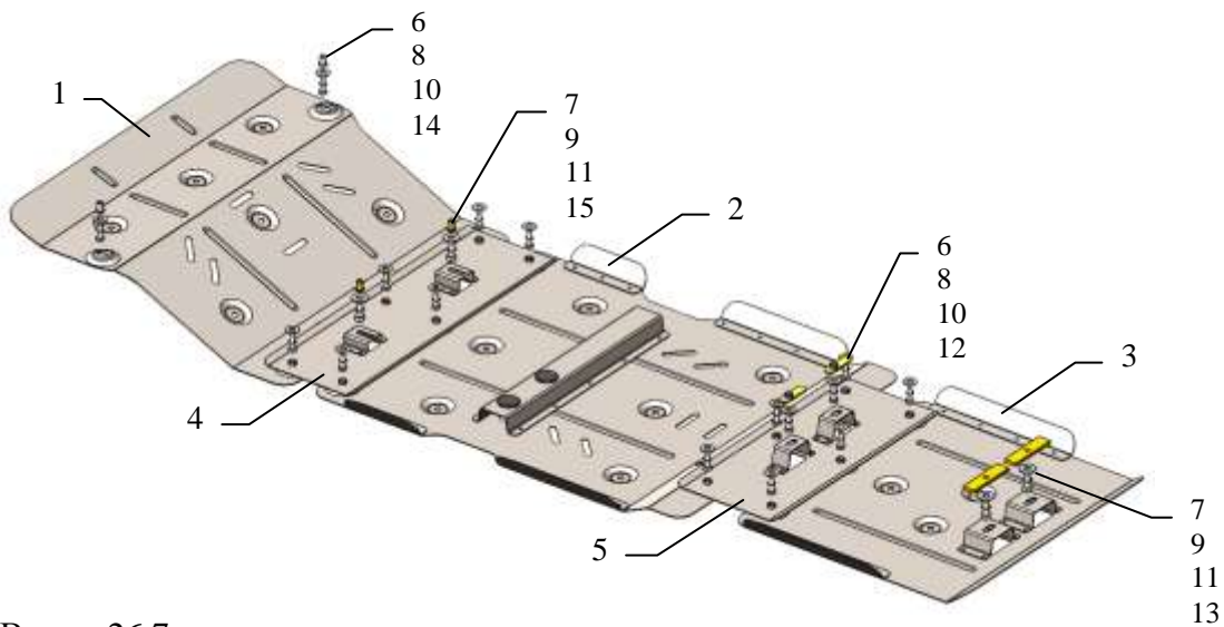
Схема збірки захиста.
