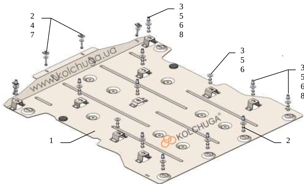
Схема сборки.
