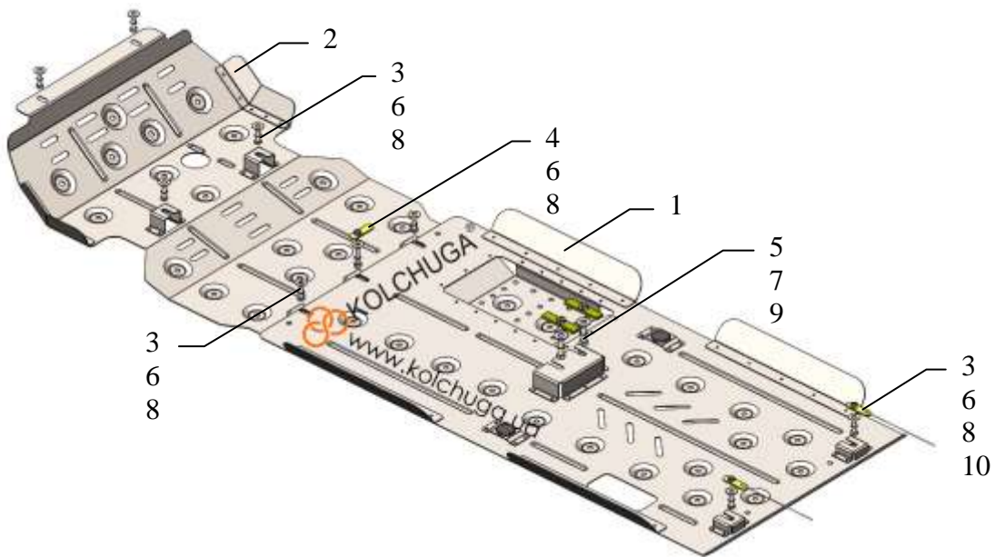
Схема сборки защиты картера и КПП.
