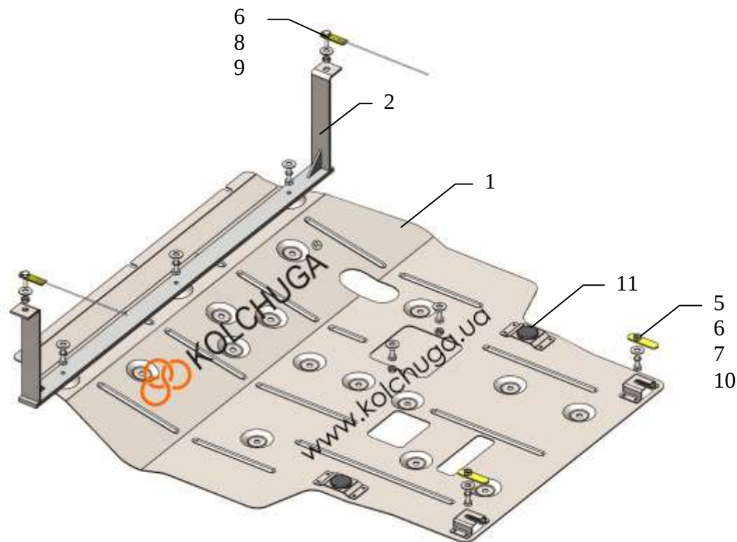
Схема установки.
