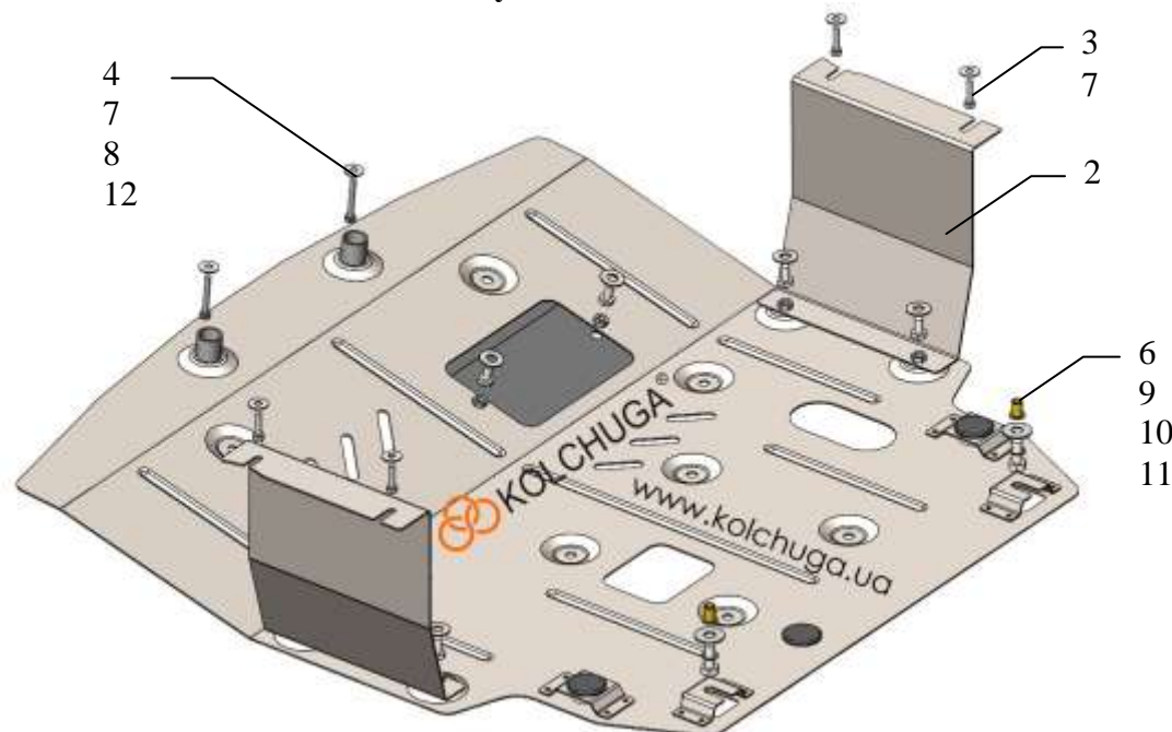
Схема установки.
