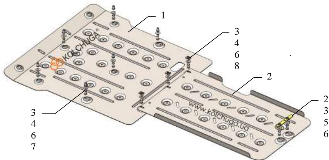
Схема сборки.
