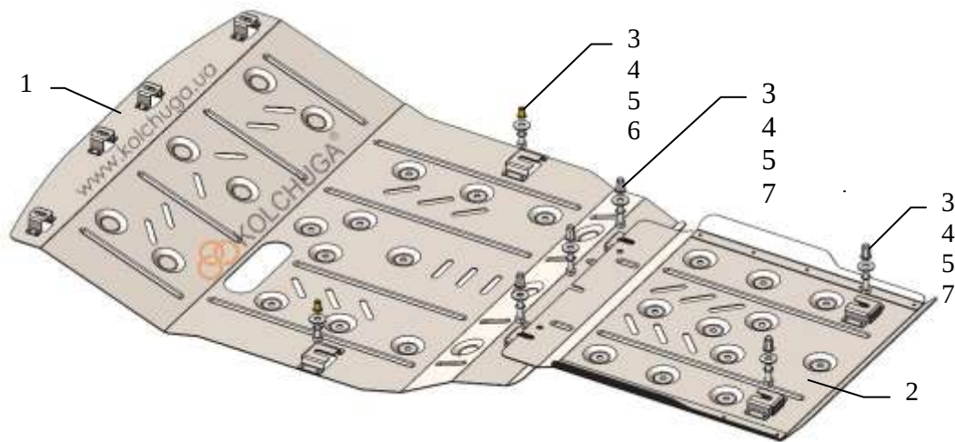
Схема сборки.
