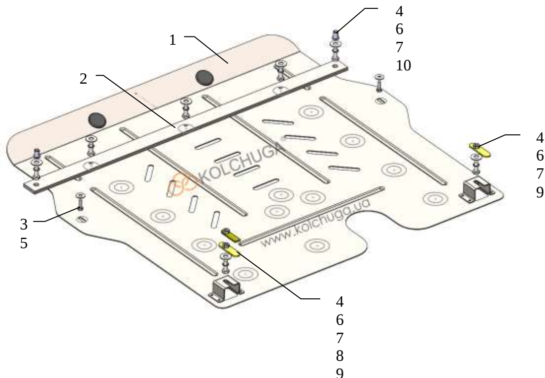
Схема установки.
