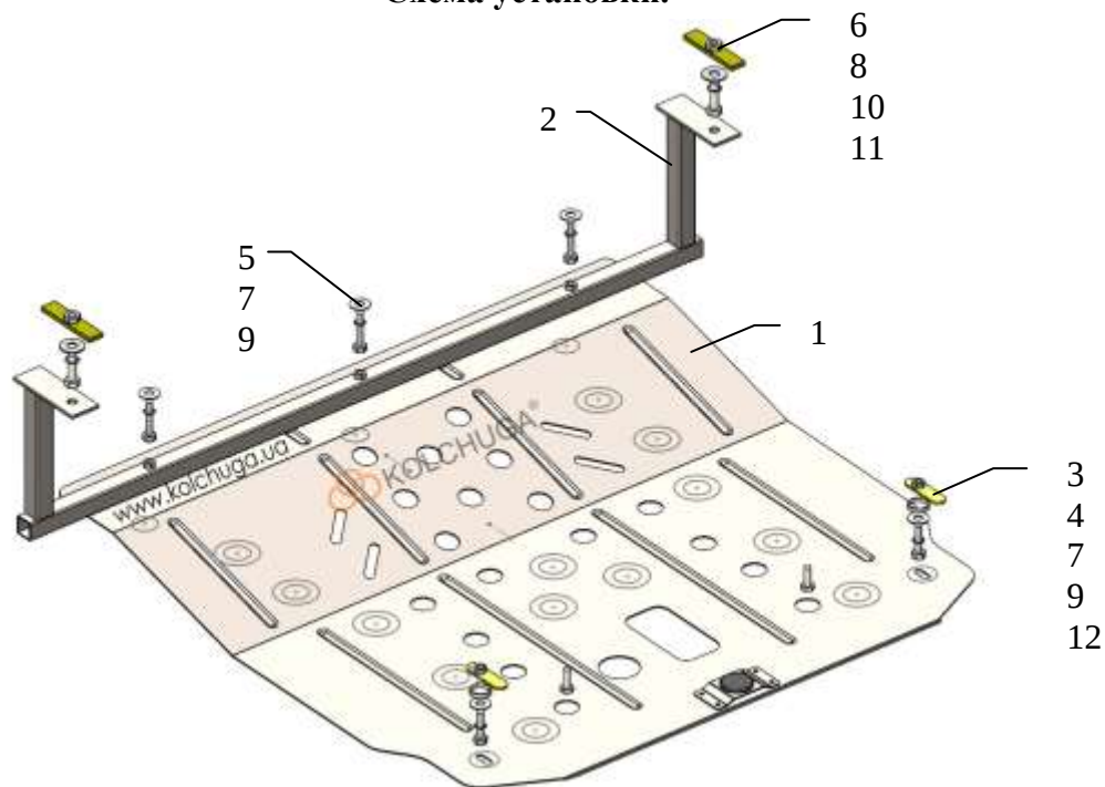
Схема установки.
