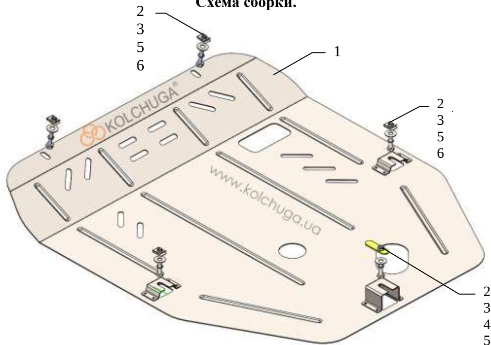
Схема сборки.
