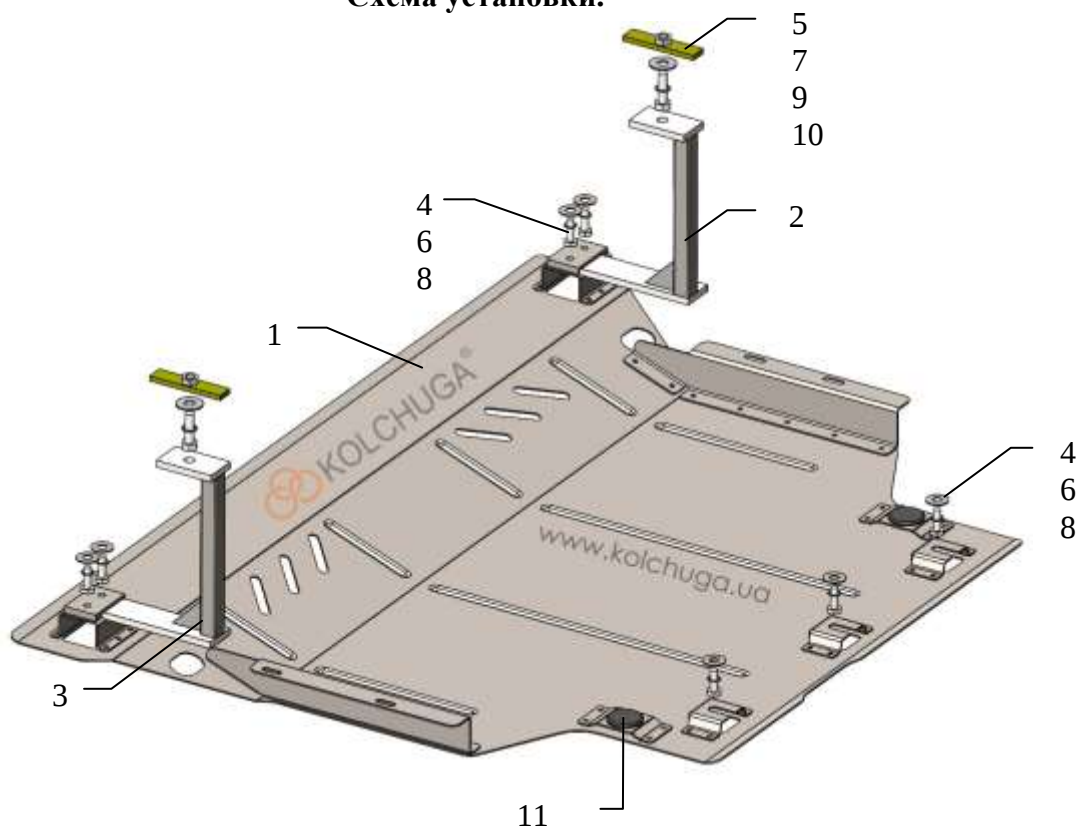
Схема установки.
