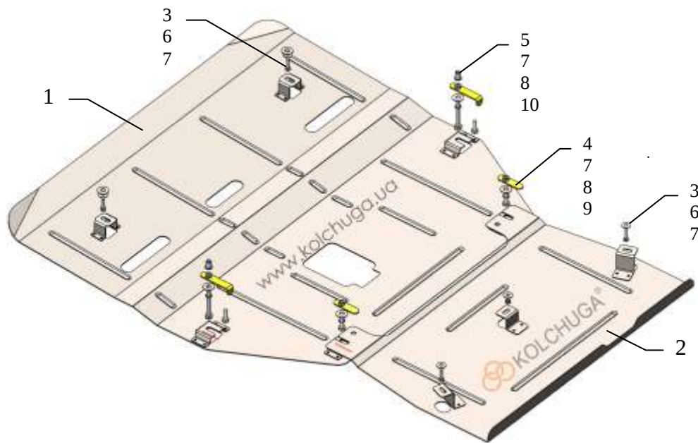
Схема сборки.
