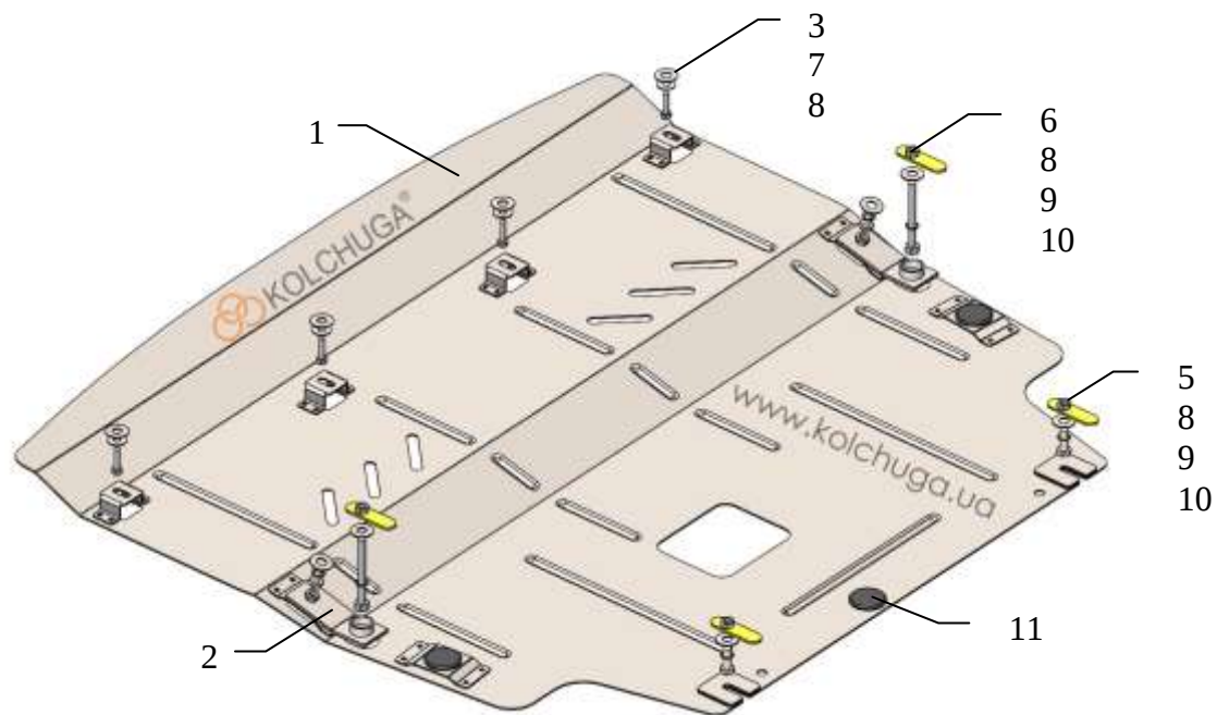
Схема установки.
