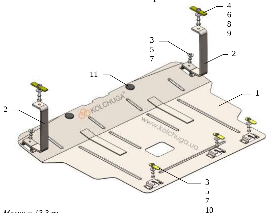
Схема сборки.
