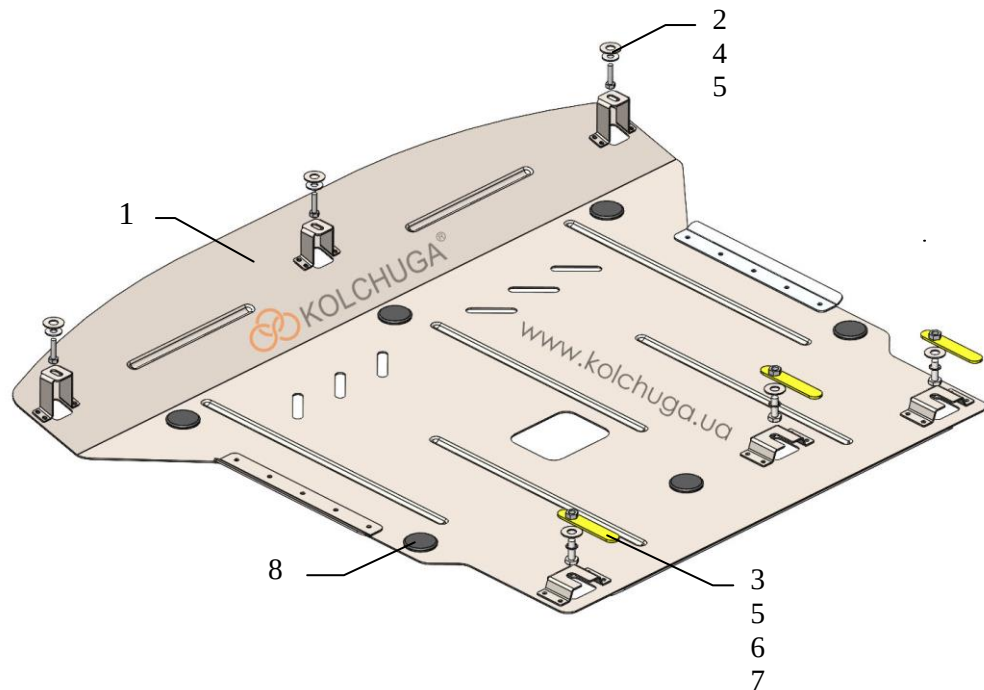
Схема сборки.
