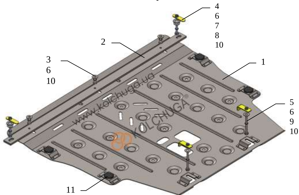
Схема сборки.
