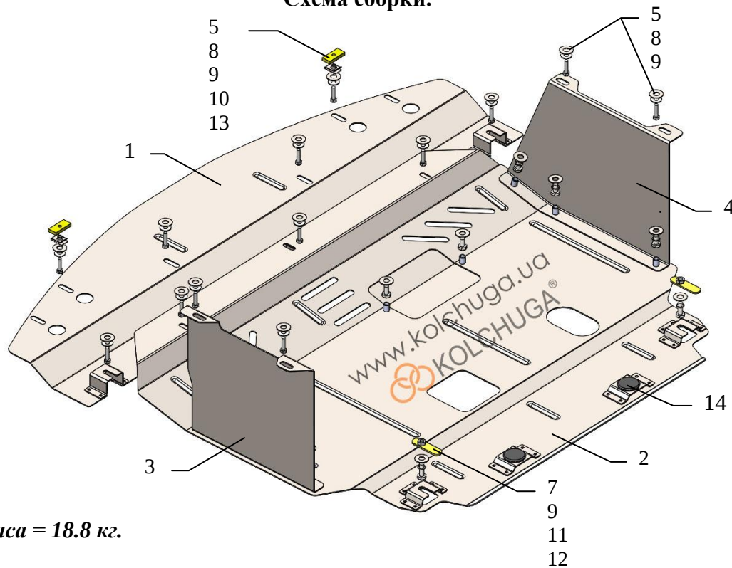
Схема сборки.
