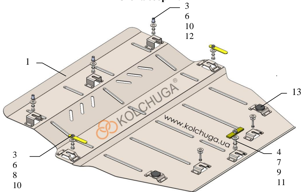
Схема сборки.
