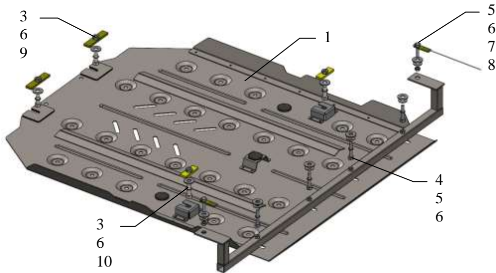
Схема сборки защиты картера и КПП.
