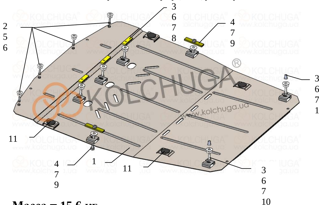
Схема сборки защиты картера, КПП, радиатора
