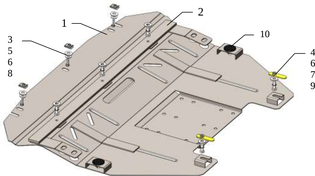
Схема сборки защиты двигателя, КПП.
