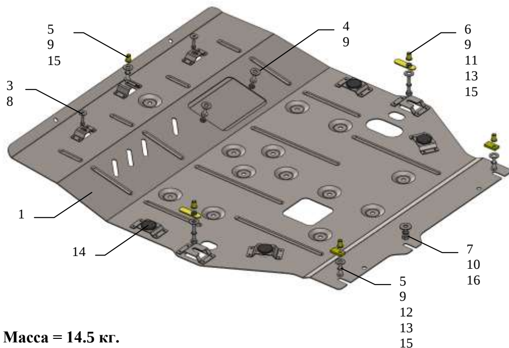
Схема сборки защиты двигателя, КПП
