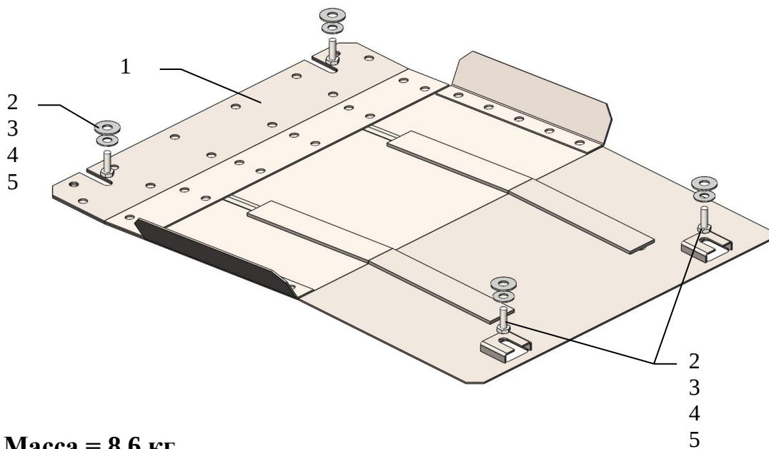
Схема сборки защиты КПП.
