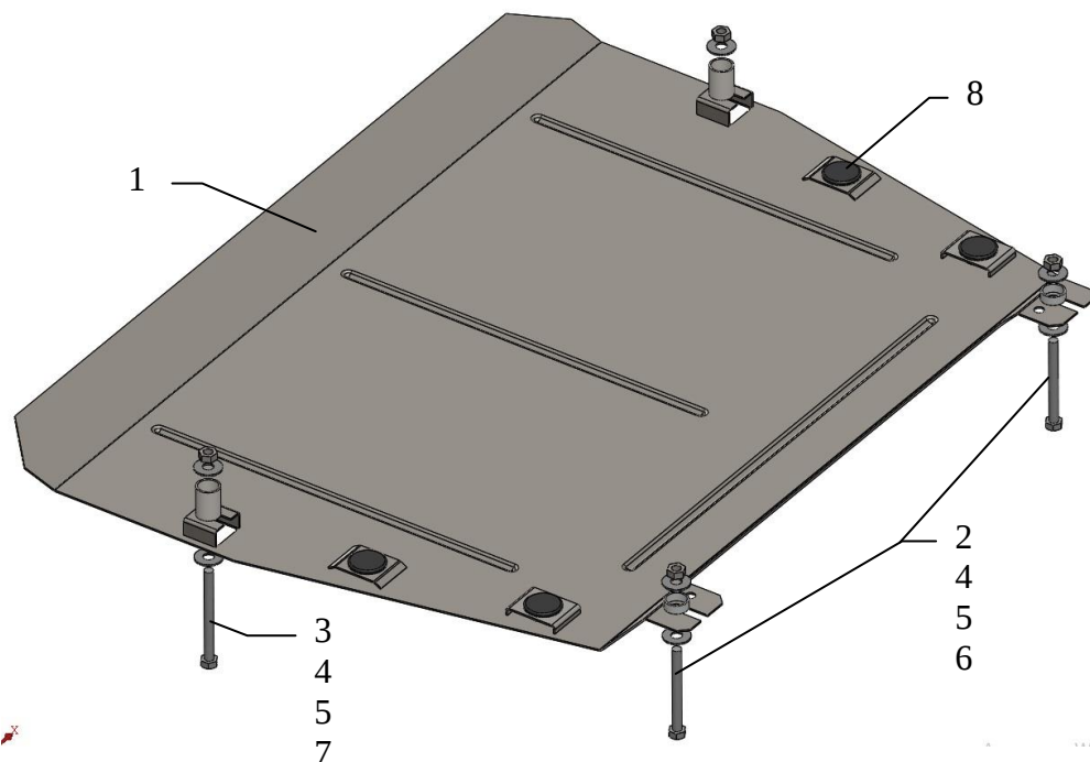
Схема сборки.
