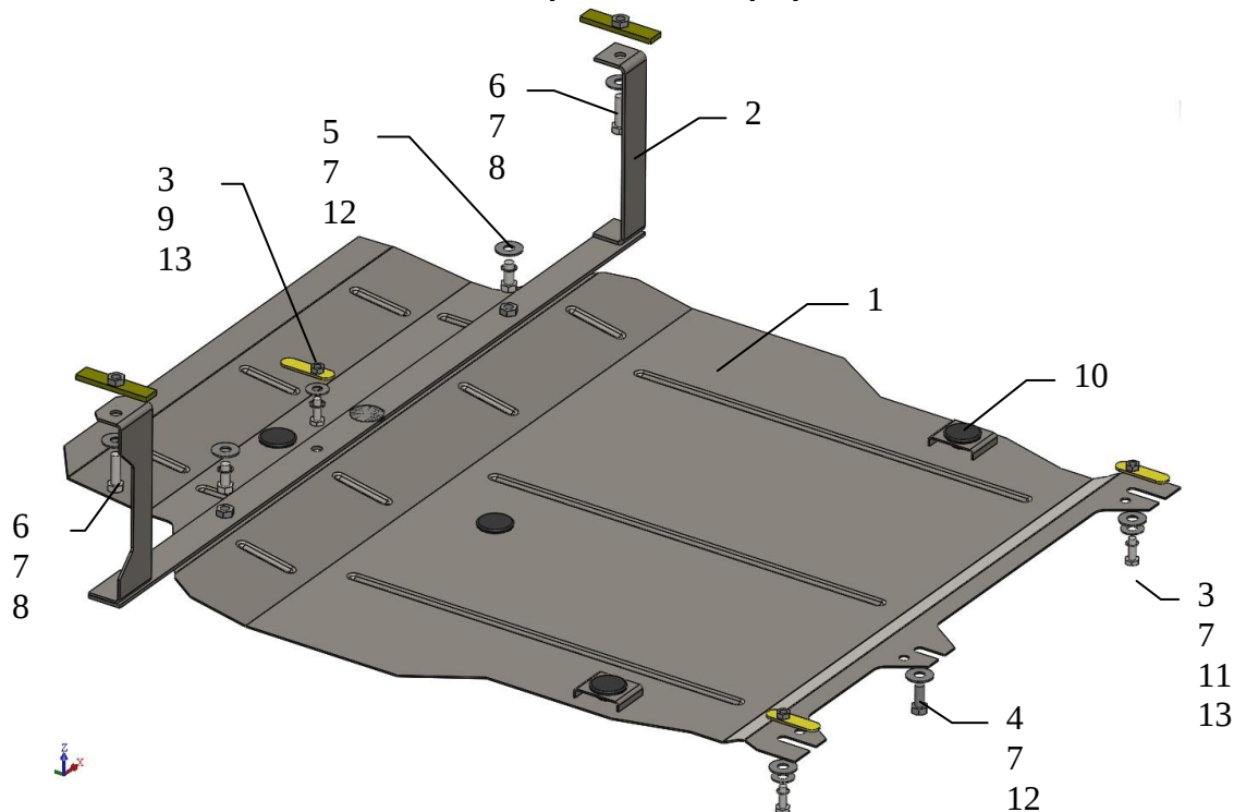
Схема сборки защиты картера .
