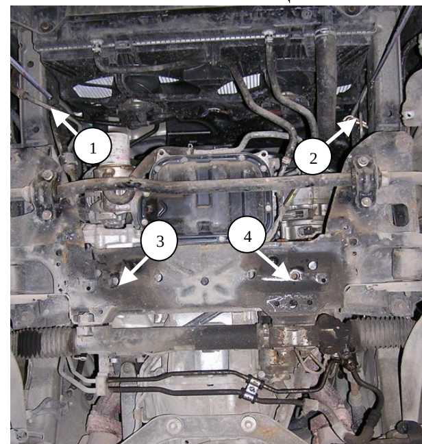
Установка защиты.
