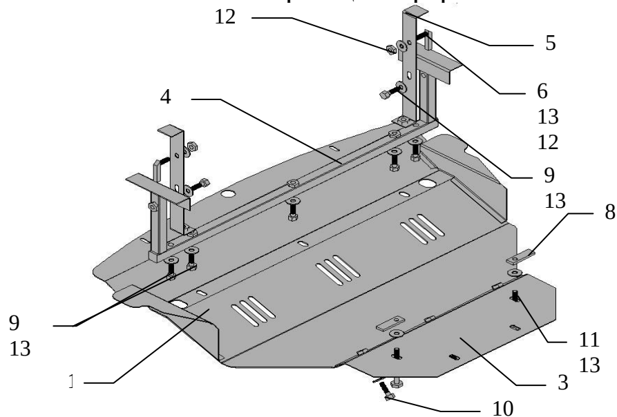
Схема сборки защиты картера
