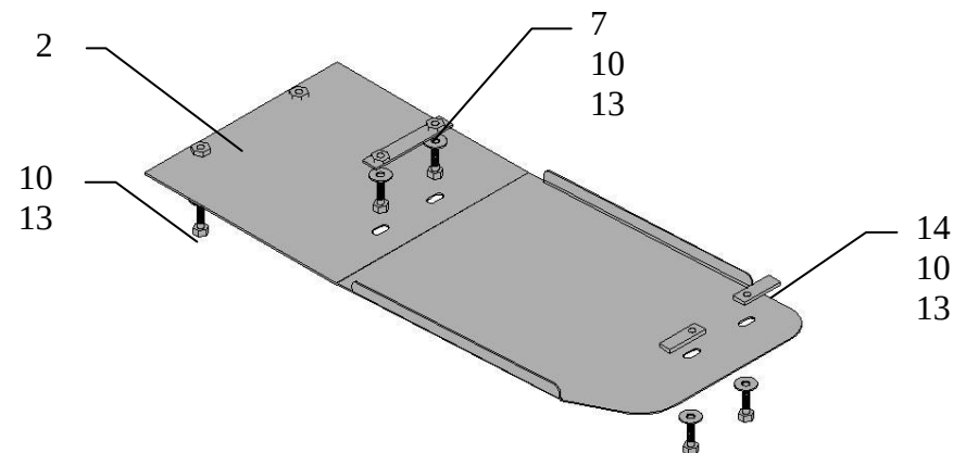
Установка защиты.
