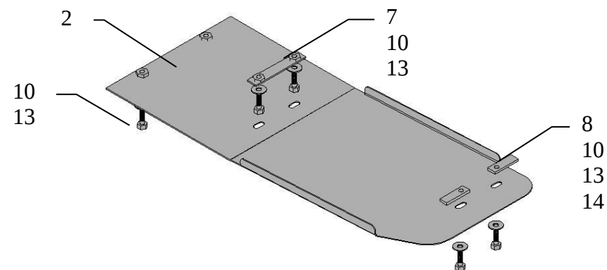
Установка защиты.
