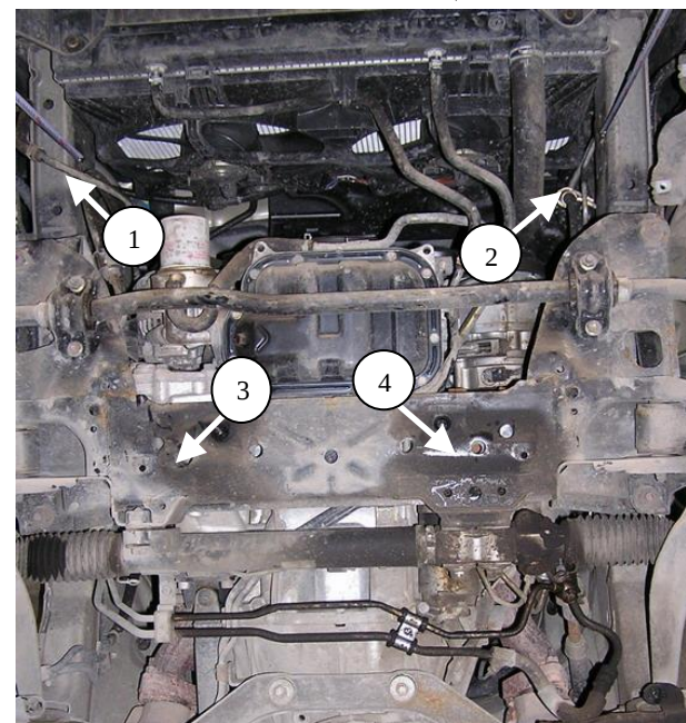
Установка защиты.
